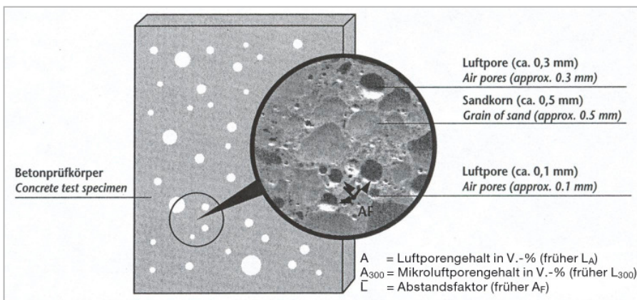
Abb. 1 Luftporenkennwerte in Beton ( A , A_{300} , \bar{L} ) aus [3]
